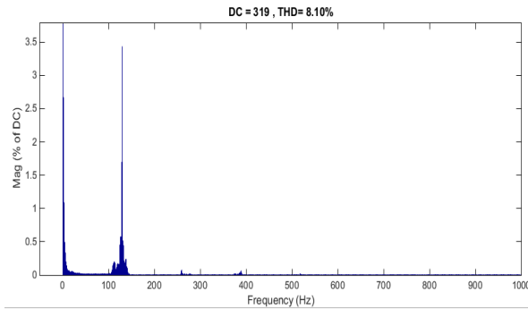
Gambar 13. Spektrum THD dari Sinyal Tegangan Beban 5 kW dengan Kontrol PID
