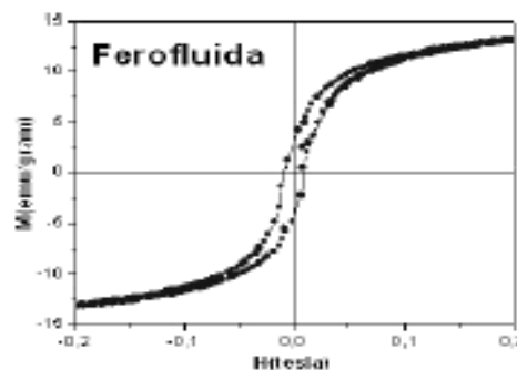
Gambar 6. Kurva histeresis untuk ferrofluida dengan Fe_3O_4 tanpa PEG-400
