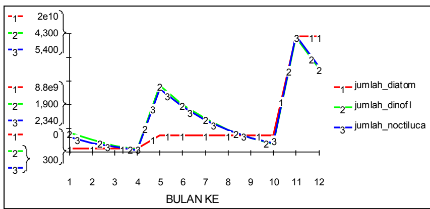
Gambar 4. Grafik waktu hasil simulasi model pertumbuhan fitoplankton untuk jumlah fitoplankton di perairan
