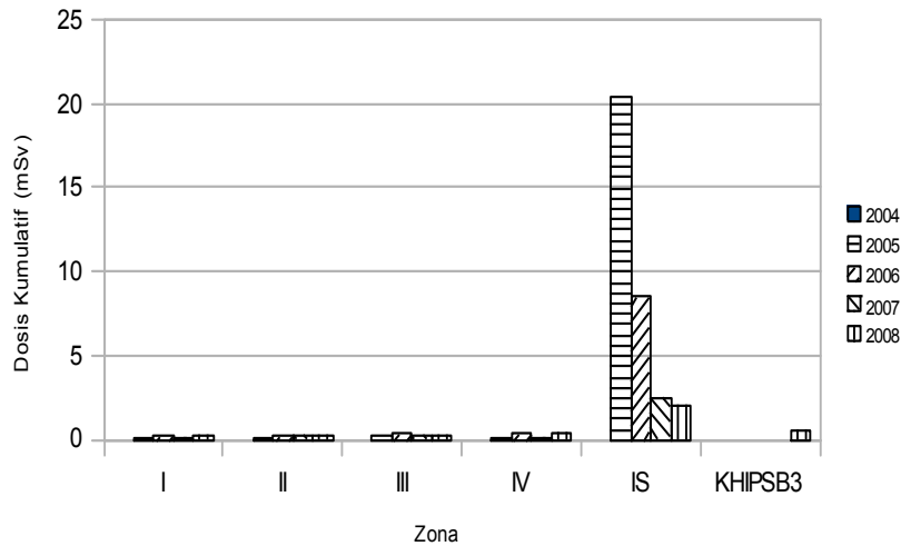
Gambar 3. Kurva Pemantauan Dosis Kumulatif daerah kerja Tahun 2005 - 2008
