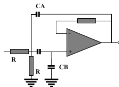
Gambar Contoh Gambar Rangkaian Band Pass Filter (BPF) Untuk Filter Aktif
