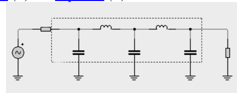
Gambar Contoh Gambar Rangkaian Low Pass Filter (LPF) Untuk Filter Pasif
