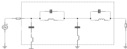
Gambar Contoh Gambar Rangkaian Band Stop Filter (BSF) Untuk Filter Pasif
