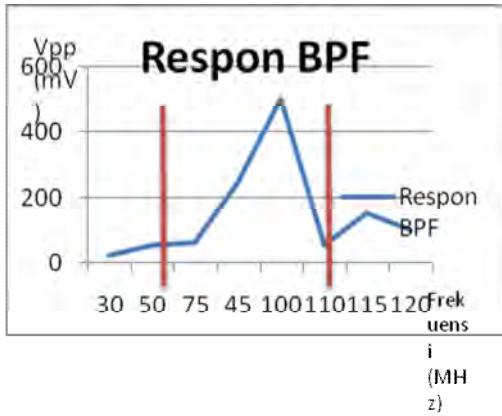
Gambar Grafik Respon BPF
