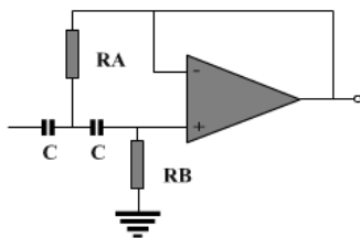
Gambar Contoh Gambar Rangkaian High Pass Filter (HPF) Untuk Filter Aktif
