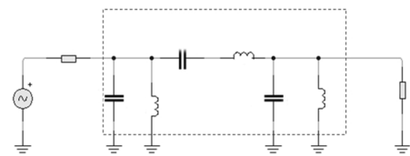
Gambar Contoh Gambar Rangkaian Band Pass Filter (BPF) Untuk Filter Pasif
