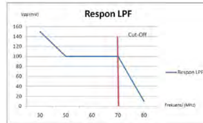
Gambar Grafik Respon LPF
