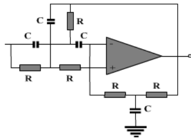
Gambar Contoh Gambar Rangkaian Band Stop Filter (BSF) Untuk Filter Aktif
