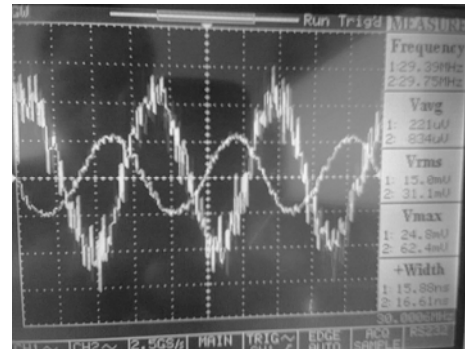
Gambar Gambar Gelombang Input dan Output Low Pass Filter
