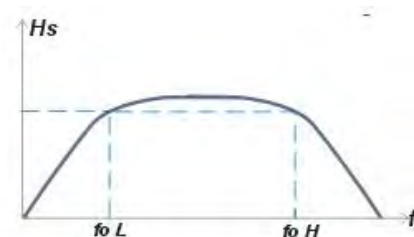
Gambar respon BPF
