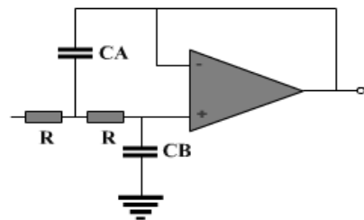
Gambar Contoh Gambar Rangkaian Low Pass Filter (LPF) Untuk Filter Aktif
