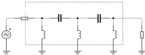
Gambar Contoh Gambar Rangkaian High Pass Filter (HPF) Untuk Filter Pasif
