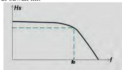
Gambar respon LPF
