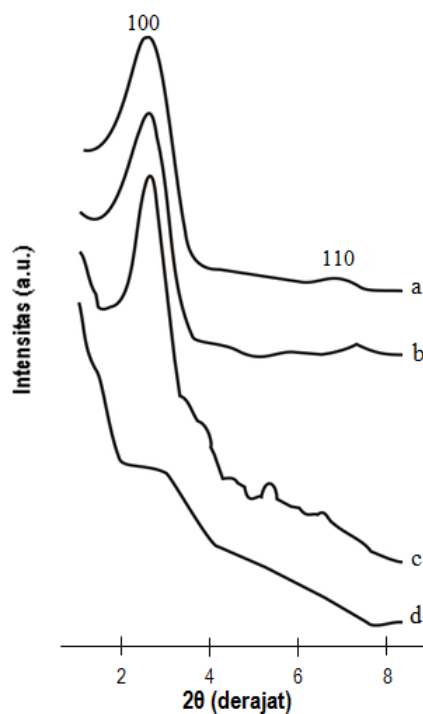
Gambar 3. Pola difraktogram XRD Fe-MCM-41-terasiliasi hasil impregnasi Fe^{3+} 0,05 M ke dalam MCM-41-terasiliasi dengan waktu kontak 8 jam pada temperatur kamar, 40, 60 dan 80 °C.
