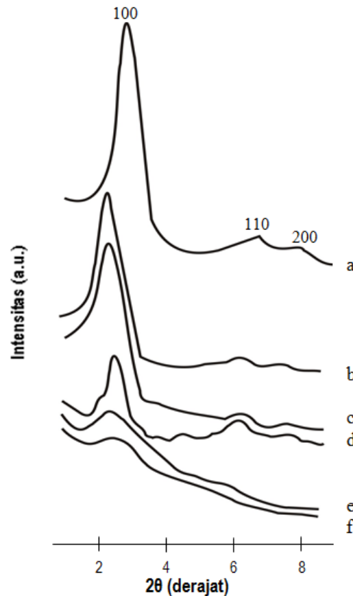
Gambar 1. Pola difraktogram MCM-41-tersililasi (a) dan Fe-MCM-41-tersililasi hasil impregnasi dengan konsentrasi \text{Fe}^{3+} masing-masing 0,01 (b), 0,05 (c), 0,10 (d), 0,5 (e), dan 1M (f).
