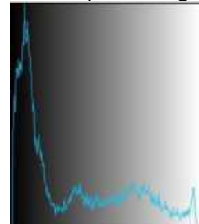
b. Histogram
