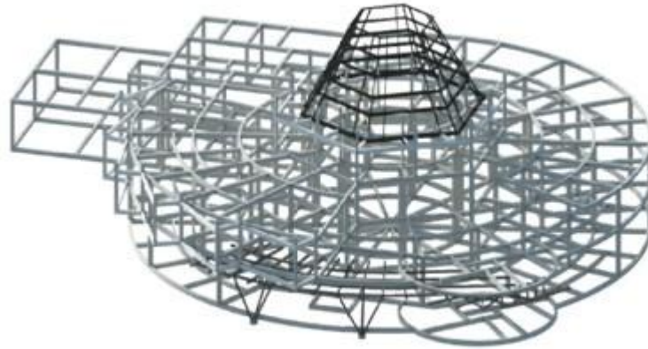
Gambar 1. Sistem Struktur
