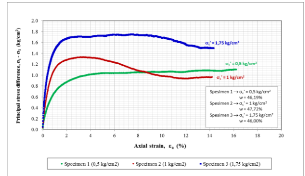
Gambar 11. Grafik hubungan tegangan regangan
