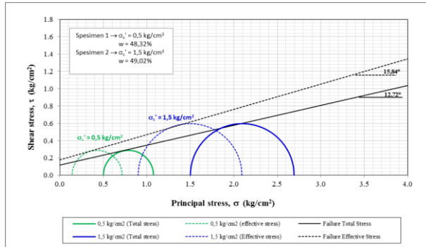
Gambar 5. Lingkaran mohr lintasan tegangan AC
