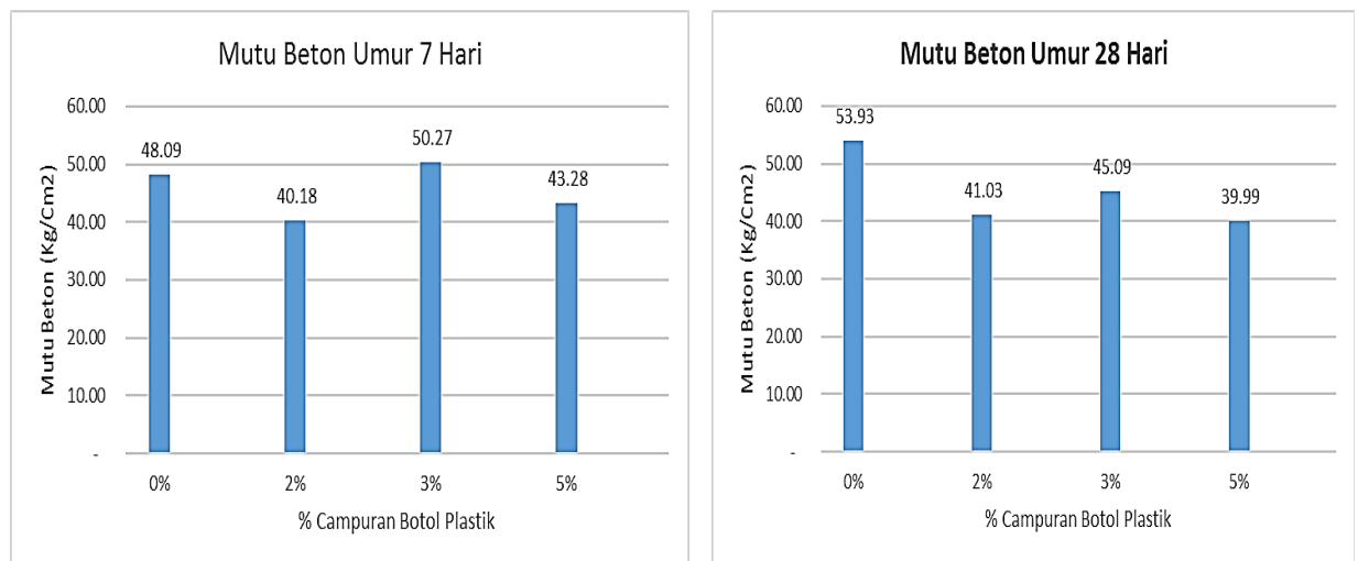
Gambar 4 : Mutu beton umur 7 dan 28 hari
