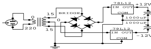
Gambar 22. Catu Daya
