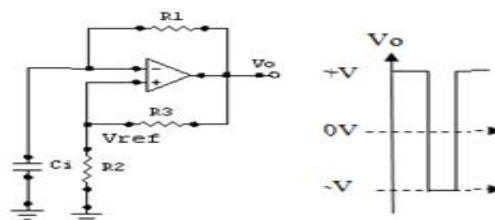
Gambar 17. Osilator Glb Kotak
