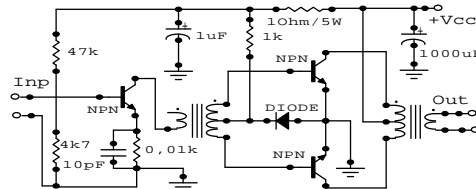
Gambar 21. Konverter
