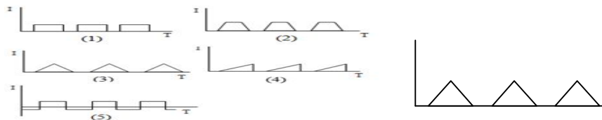
Gambar 11. Modifikasi sinyal impuls (J.F Gabriel, 1996: 249).
