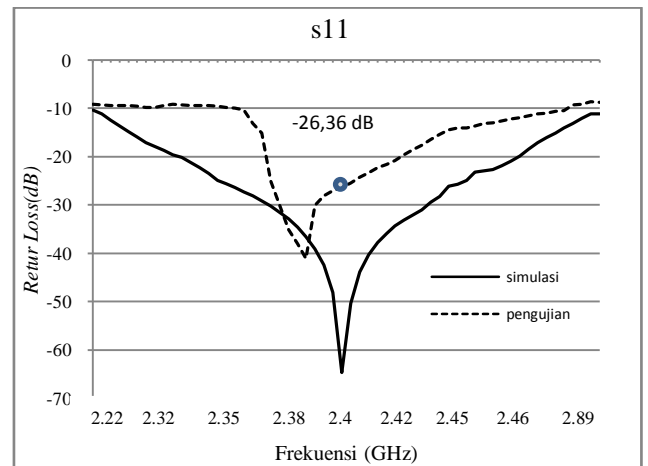
Gambar 10. Return loss antenna hasil pengujian dan simulai
