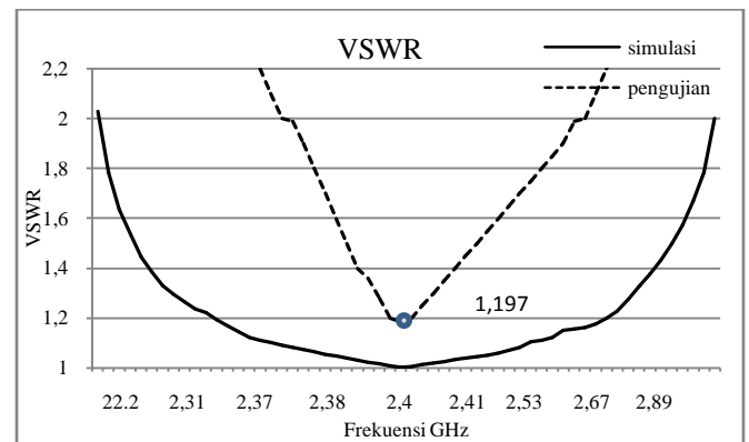
Gambar 11. VSWR antenna hasil pengujian dan simulai
