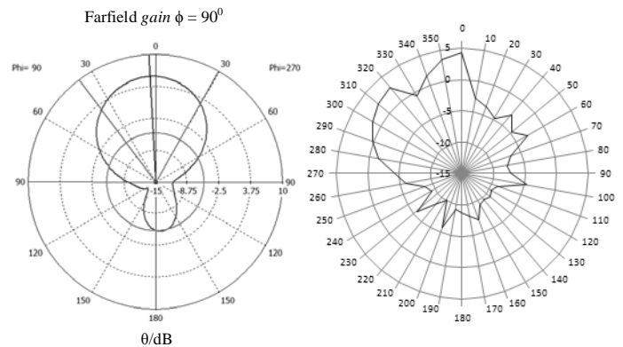
Gambar 15. Pola radiasi antenna loop (a) hasil simulasi, (b) hasil pengujian
