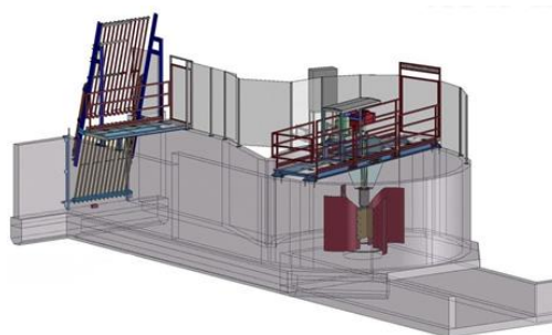
Gambar 2.1 Tubin Vortex (Pusaran Air)
