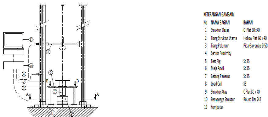
Gambar 6. Perangkat Alat Uji Impact Jatuh Bebas
