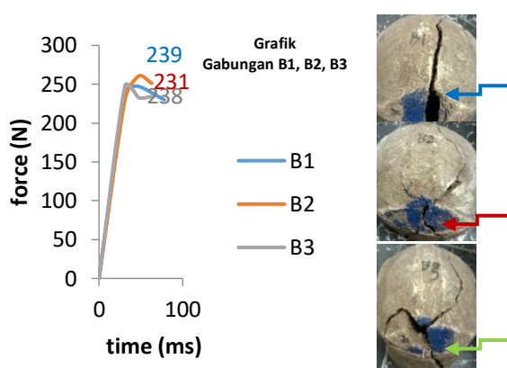
Gambar 10. Grafik gabungan gaya vs waktu impak ketinggian 1 meter.
