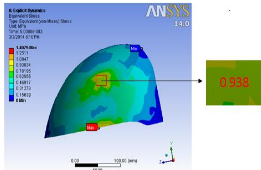
Gambar 2. Distribusi tegangan pada sisi kiri helm sepeda
