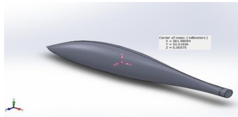
Gambar 26. Pusat massa pada badan pesawat tanpa awak secara utuh
