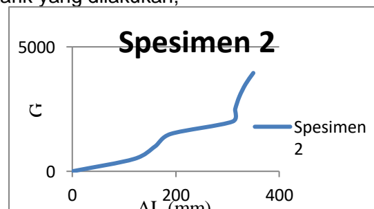
Gambar 16. Grafik spesimen 2
