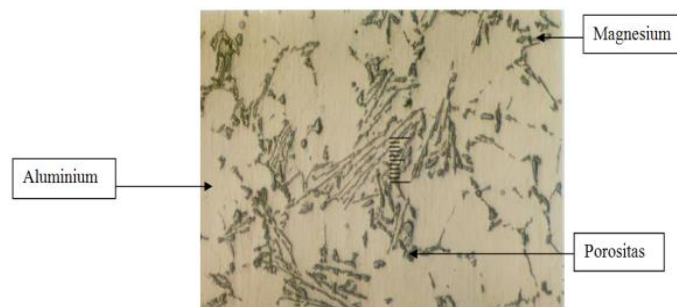
Gambar 5 Mikrostruktur paduan aluminium yang tidak distempering
