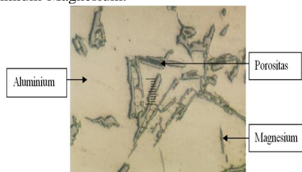
Gambar 8 Mikrostruktur paduan aluminium ditempering Suhu 400^{\circ}\text{C}
