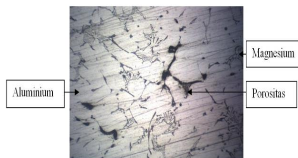
Gambar 7 Mikrostruktur paduan aluminium ditempering Suhu 300^{\circ}\text{C}
