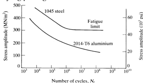
Gambar 1 Kurva S-N
