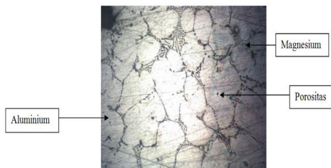
Gambar 6 Mikrostruktur paduan aluminium ditempering Suhu 200 0 C
