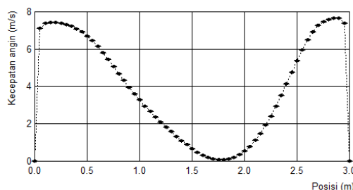
Gambar 6. Grafik kecepatan angin pada sisi outlet
