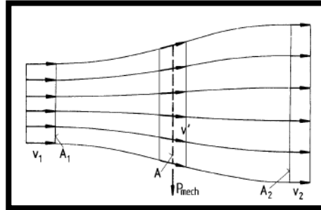
Gambar 2. Kondisi aliran udara pada proses pengambilan energi mekanik menurut teori momentum elementer [3]
