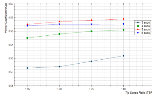
Gambar 9. Grafik tip speed ratio vs koefisien daya untuk semua jumlah sudu
