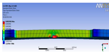
Gambar 10 Simulasi regangan
