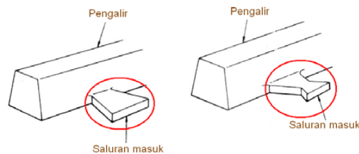
Gambar 2. Saluran masuk
