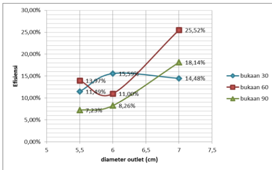
Gambar 4.10 grafik outlet vs efisiensi pada Sudu I Setelah menganalisa terhadap outlet maka dianalisa terhadap debit air masuk (bukaan katup). Efisiensi maksimal mencapai 25,52% di bukaan 60° pada sudu I.
