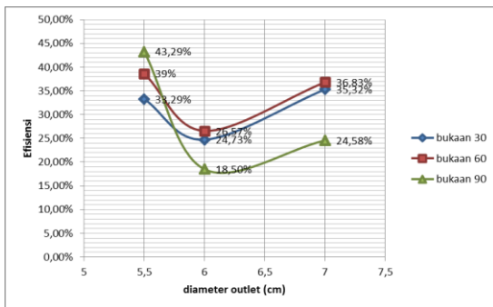
Gambar 4.11 grafik outlet vs efisiensi pada sudu III Sedangkan dengan cara yang sama, di sudu III efisiensi maksimal dapat mencapai 43,29% di bukaan 90°.
