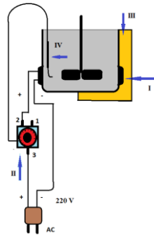
Gambar 4.2 Rangkaian Listrik
