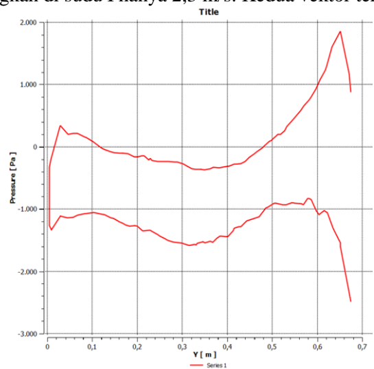
Gambar 4.5 grafik distribusi tekanan pada sudu I
