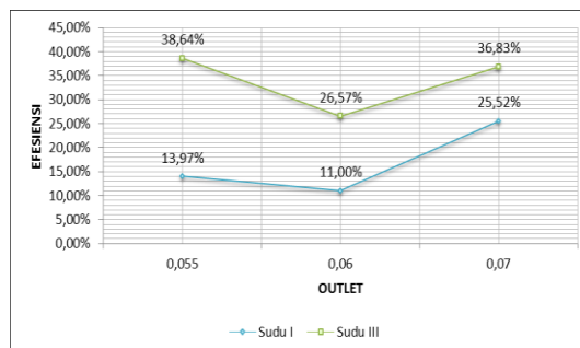
Gambar 4.8 grafik outlet vs efisiensi pada bukaan 60° Efisiensi maksimal mencapai 38,64% di outlet 5 cm.
