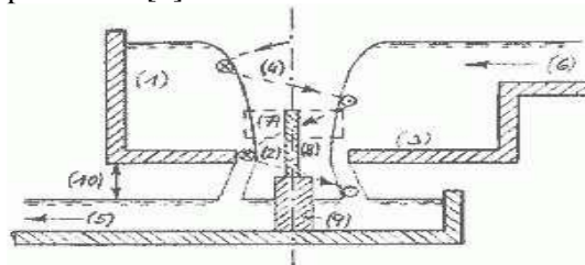
Gambar 2.4 skema aliran vortex
