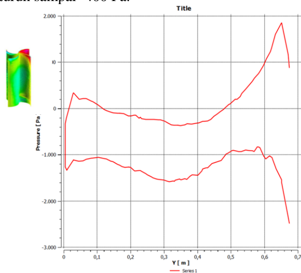
Gambar 4.6 grafik distribusi tekanan pada sudu III
