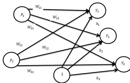
Gambar 1. Arsitektur Jaringan Self Organizing Map
