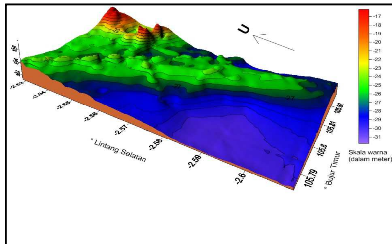
Gambar 4. Morfologi Kedalaman Dasar Laut (Batimetri) Daerah Penelitian, Selat Bangka dalam Bentuk 3D.
