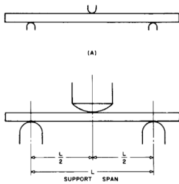
Gambar 2. Skema Uji Bending
