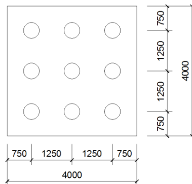
Gambar 10. Pondasi P1
