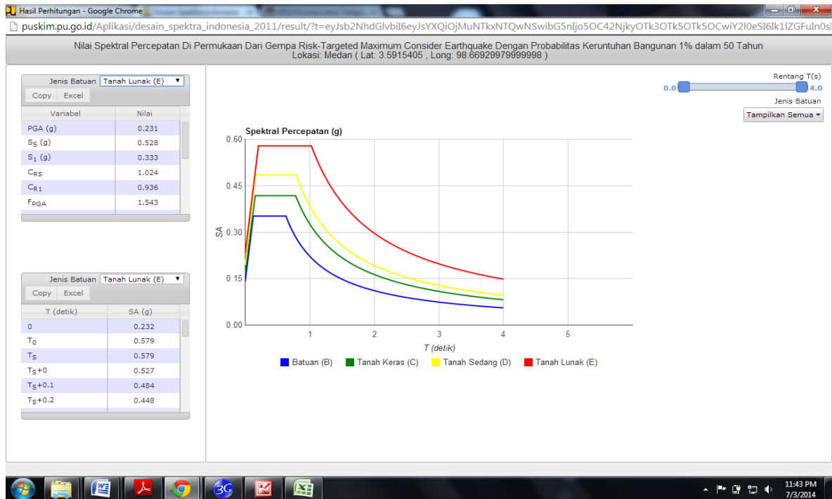
Sumber : puskim.pu.go.id/Aplikasi/desain_spektra_indonesia_2011
