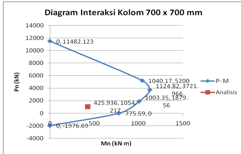
Gambar 9. Diagram Interaksi M- P Kolom Menggunakan Perhitungan Manual
