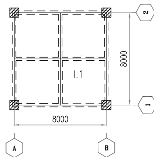
Gambar 5. Plat Lantai Tipe I.1
