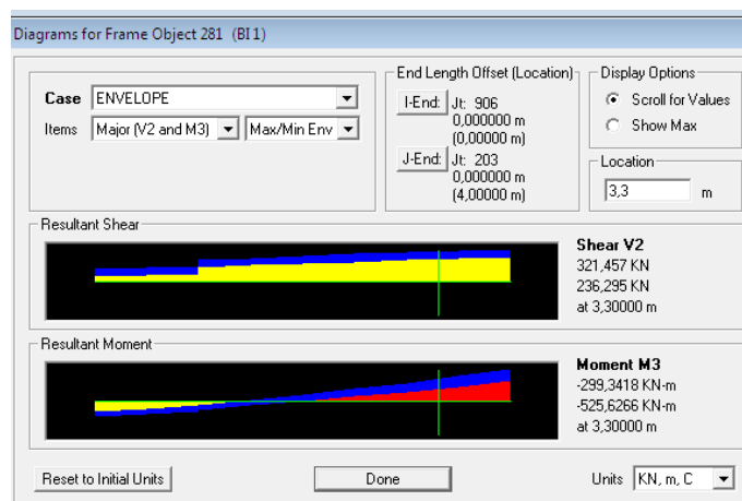
Gambar 8. Diagram Momen Tumpuan Balok Induk
