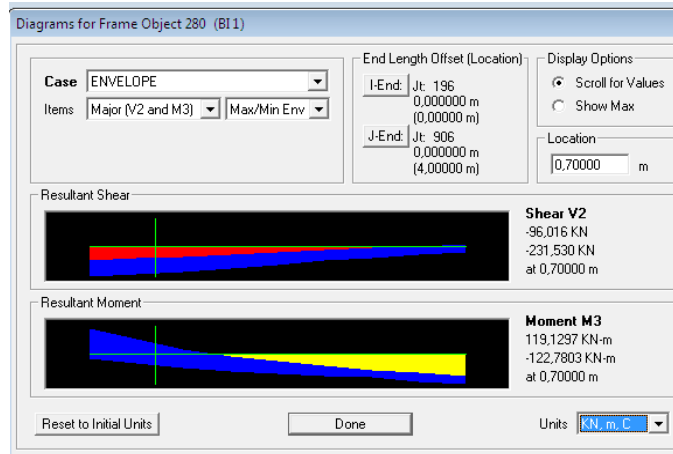
Gambar 6. Diagram Momen Tumpuan Balok Induk
