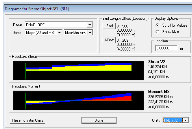
Gambar 7. Diagram Momen Lapangan Balok Induk
