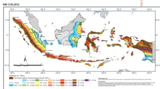
Gambar 3 - S_s Gempa maksimum yang dipertimbangkan risiko tertarget ( MCE_d ) kelas situs SD
