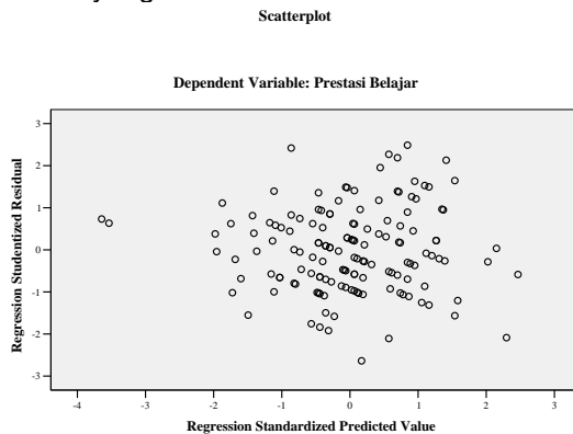
Gambar 2 Gambar Penyebaran Plot Uji Linearitas
