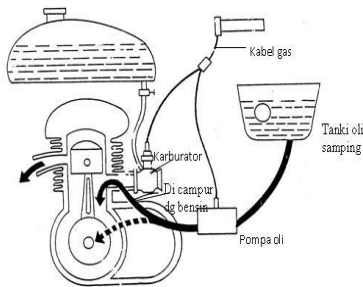
Gambar 2 : Sistem Pelumasan Autolube
