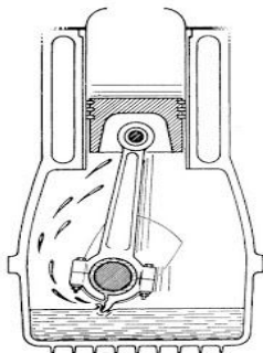
Gambar 3 : Sistem Pelumasan Percik
