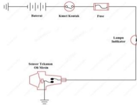
Gambar 9: Sensor Tekanan Oli
