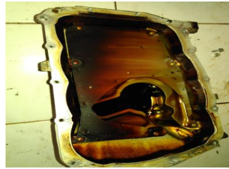
Gambar 15 : Pembongkaran dan pengecekan bak penampung oli
