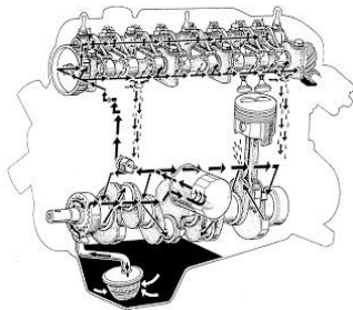
Gambar 4 : Sistem Pelumasan Tekan
