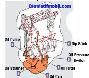
Gambar 11 : Cara Kerja Sistem Pelumasan
