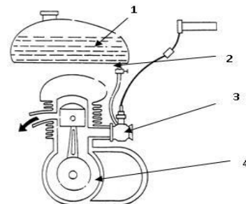
Gambar 1 : Sistem Pelumasan Campur
