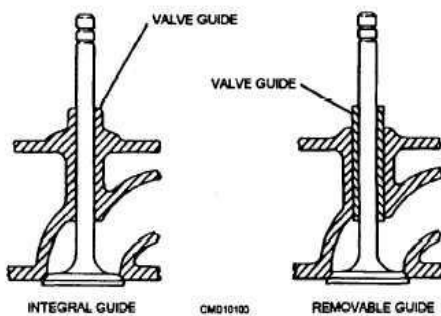
Gambar 8: Penghantar Katup
