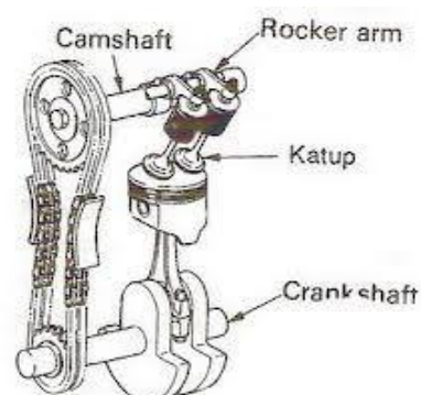
Gambar 2: Mekanisme Katup Tipe OHC
