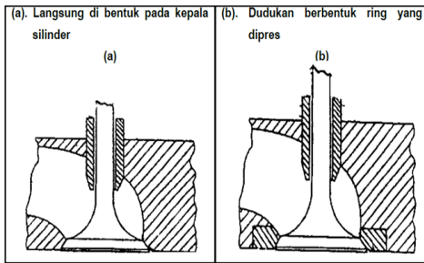
Gambar 7: Dudukan Katup
