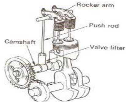
Gambar 1: Mekanisme Katup Tipe OHV
