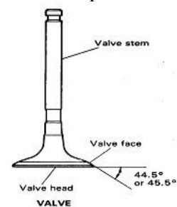
Gambar 6: Katup
