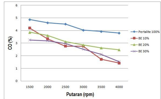
Gambar 6. Perbandingan Hubungan Kadar CO terhadap Putaran Mesin dengan Menggunakan Variasi Bahan Bakar
