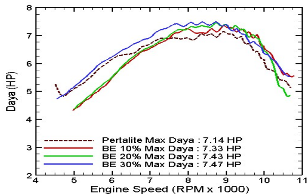
Gambar 3. Hubungan Daya terhadap Putaran Mesin dengan Menggunakan Variasi Bahan Bakar Bioetanol
