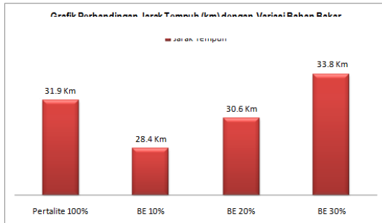
Gambar 5. Perbandingan Jarak Tempuh dengan Variasi Bahan Bakar
