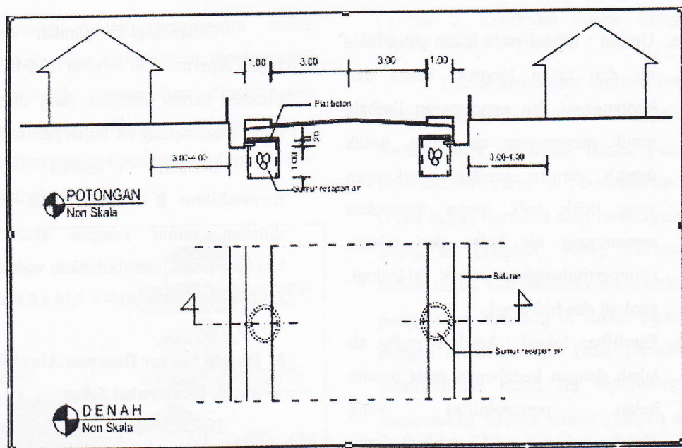
Gambar 4. Resapan Air pada Konstruksi Jalan
