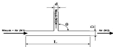
Gambar 1. Model sederhana dari T-junction
