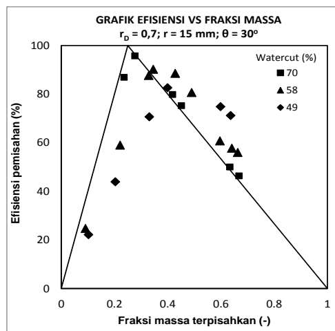
Gambar 10. Efisiensi pemisahan fase pada sudut kemiringan 30°
