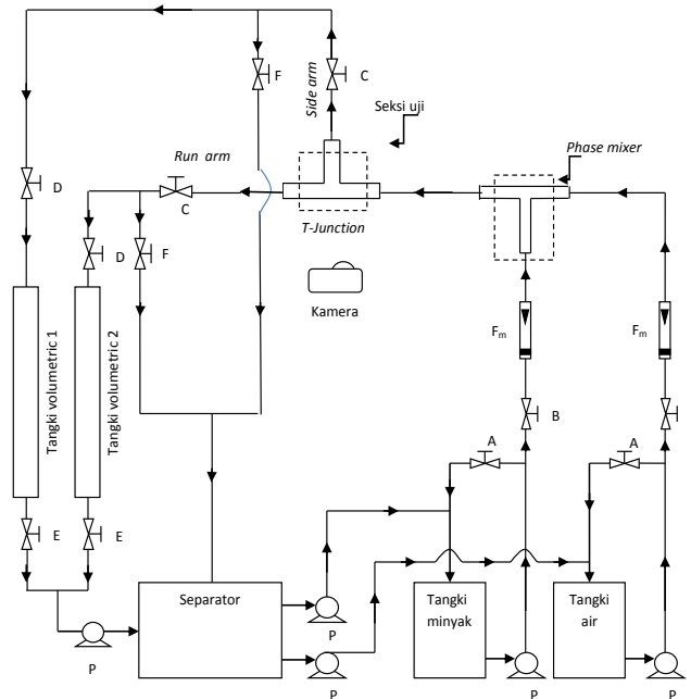
Gambar 5. Skematik diagram eksperimental
