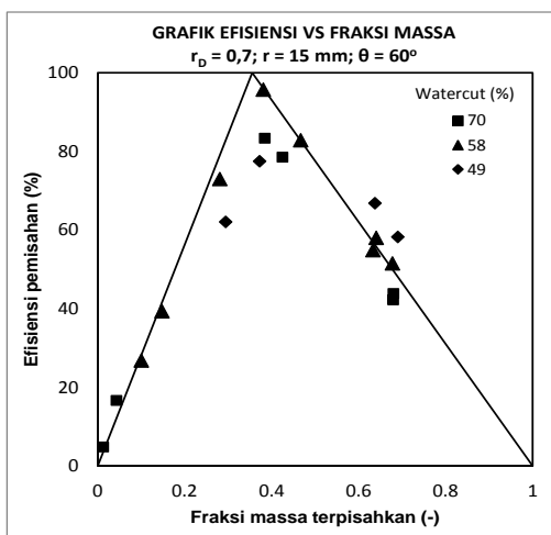
Gambar 8. Efisiensi pemisahan fase pada sudut kemiringan 60°
