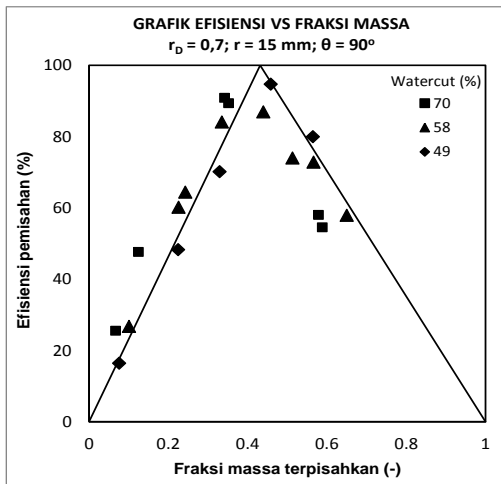
Gambar 6. Efisiensi pemisahan fase pada sudut kemiringan 90°
