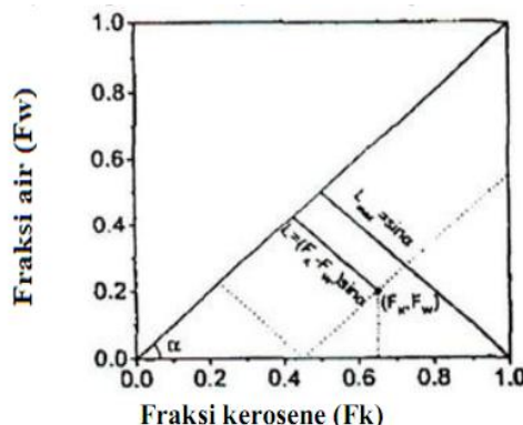
Gambar 3. Kriteria untuk menunjukkan pemisahan fase di T-junction [9].
