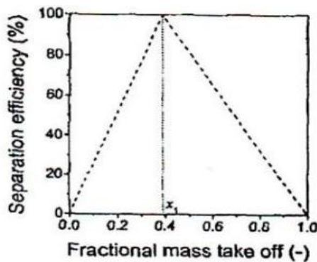
Gambar 4. Metode penyajian efisiensi pemisahan pemisahan ideal T-junction [9].
