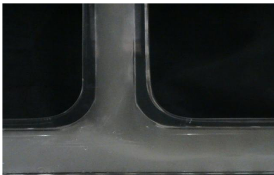
Gambar 14. Visualisasialiran (3L-2) untuk kondisi terbaik pada gambar 7
