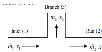
Gambar 2. Parameter aliran dua fase di T-junction [9].
