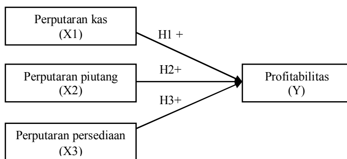
Gambar 1 : Desain penelitian
