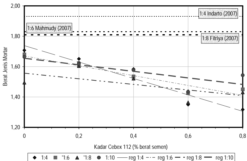
Gambar 2. Hubungan kadar Cebex 112 dengan berat jenis mortar limbah bata
