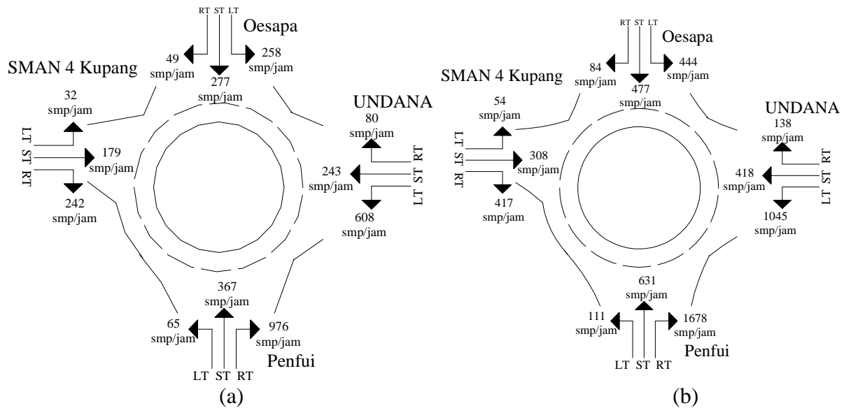
Gambar 3.(a) Arus Lalu-lintas Pada Tahun 2017, (b) Arus Lalu-lintas Hasil Proyeksi Pada Umur Rencana 10 Tahun (Tahun 2027)
