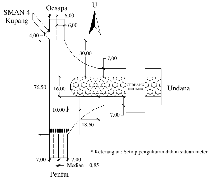
Gambar 2. Geometrik Simpang Eksisting
