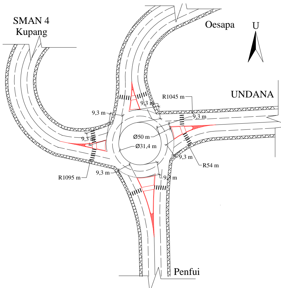
Gambar 3. Layout Hasil Desain Bundaran
