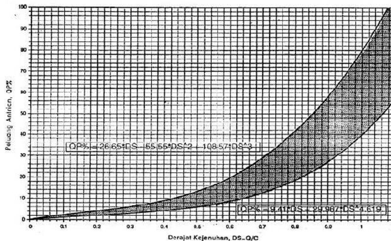
Gambar 1. Peluang Antrian vs Derajat Kejenuhan (QP Vs DS) (DEPHUB, Bina Marga)
