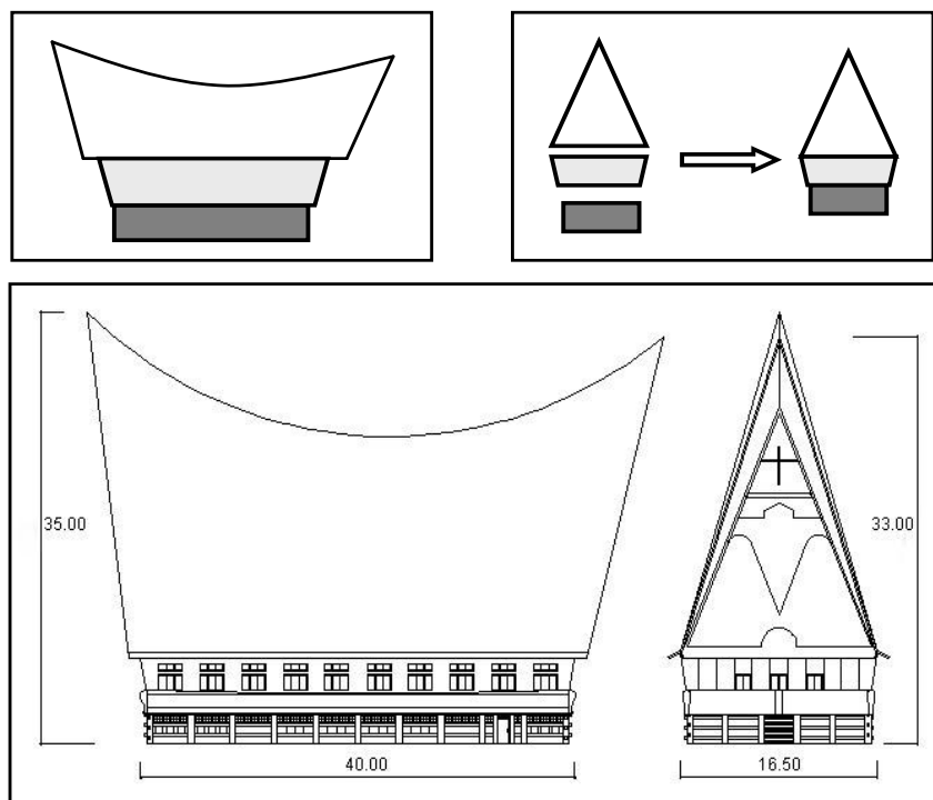
Gambar 3. Tampak samping dan tampak depan bangunan GKIP
