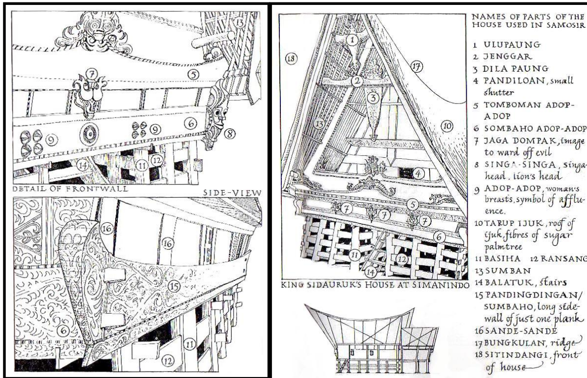
Gambar 2. Gorga rumah Batak dan bagian-bagiannya (Joosten, 1992: 80)
