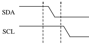
Gambar 2. Timing Diagram Untuk START
