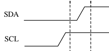
Gambar 3. Timing Diagram Untuk STOP
