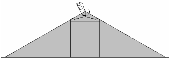
Gambar 9. Metode Sudut Proteksi dengan \alpha = 60^0 pada Gedung W UK Petra (Tampak Depan)
