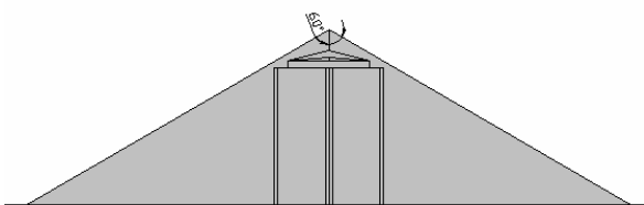
Gambar 10. Metode Sudut Proteksi dengan \alpha = 60^0 pada Gedung W UK Petra (Tampak Samping)
