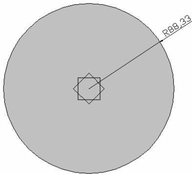
Gambar 8. Metode Sudut Proteksi dengan \alpha = 60^0 pada Gedung W UK Petra (Tampak Atas)
