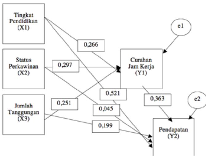
Gambar 2. Diagram Analisis Jalur Penelitian
