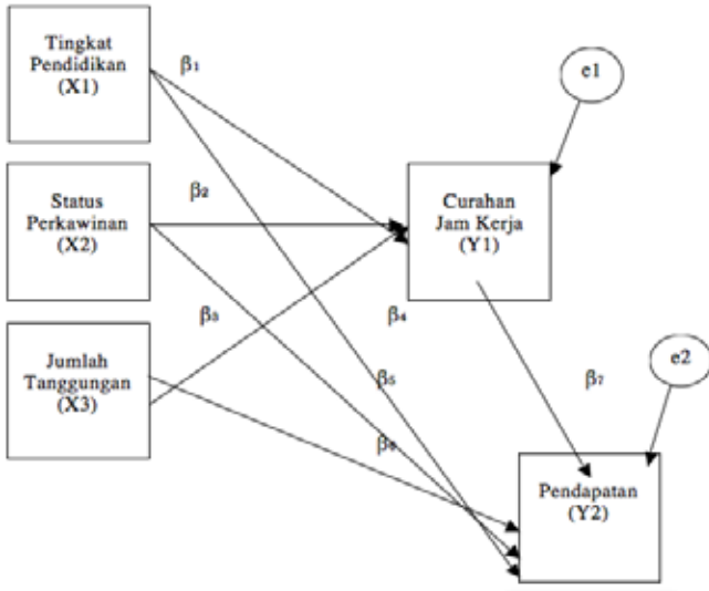
Gambar 1. Desain Penelitian Analisis Jalur
