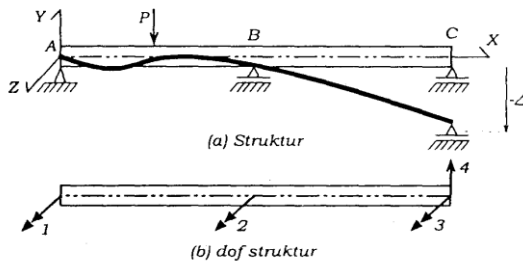
Gambar 2. Struktur di bawah pengaruh amblasannya dan beban luar
