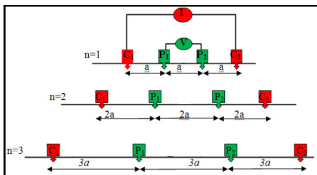
Gambar2. Konfigurasi Wenner
