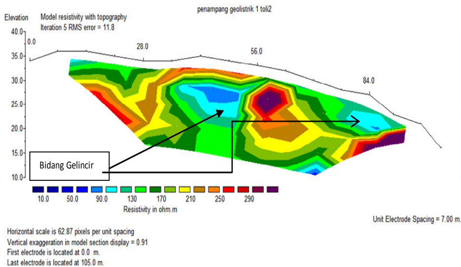
Gambar 4. Penampang topografi geolistrik lintasan 1
