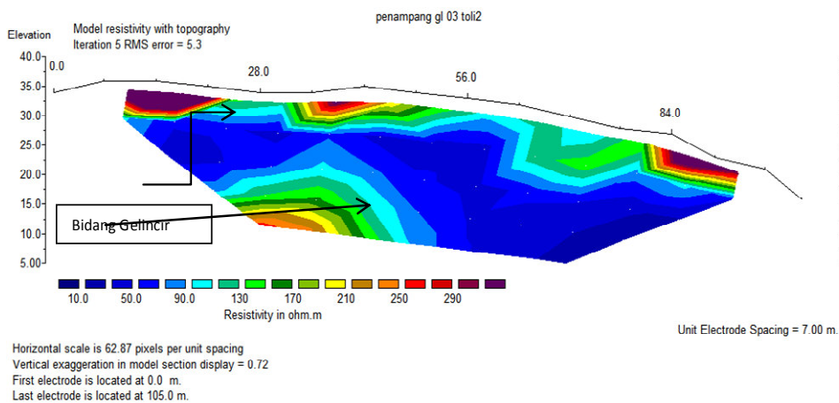
Gambar 6. Penampang geolistrik lintasan Geolistrik 3 KM 513
