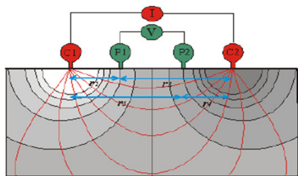
Gambar 1. Prinsip pengukuran geolistrik hambatan jenis
