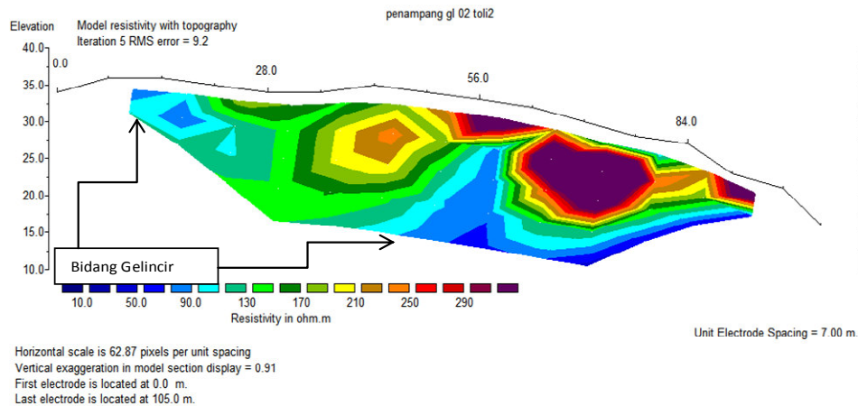
Gambar 5. Penampang geolistrik lintasan Geolistrik 3 KM 513
