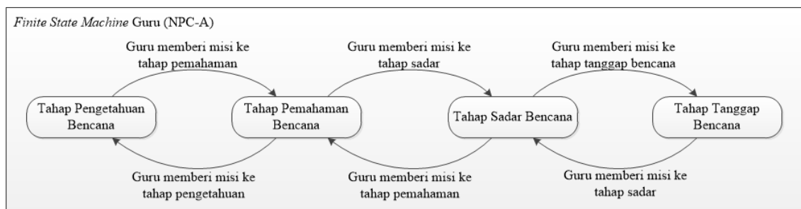
Gambar 5. FSM guru (NPC-A)
