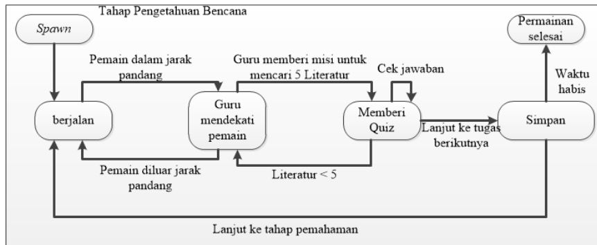
Gambar 6. FSM guru (NPC-A) untuk tahap pengetahuan bencana
