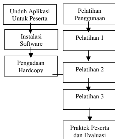
Gambar 10. Rancangan Penelitian
