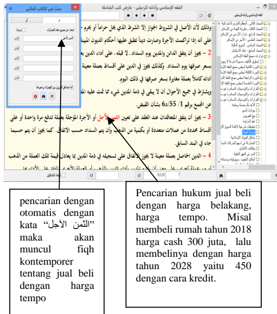
Gambar 7. Gambaran Implementasi
