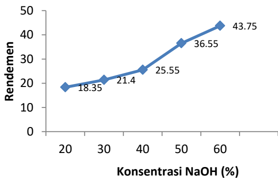
Gambar 1. Rendemen O-KMK pada berbagai konsentrasi NaOH
