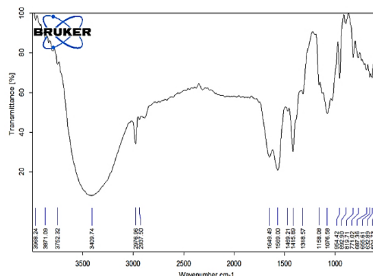
Gambar 8. Hasil analisis FTIR pada suhu 30^{\circ}\text{C}
