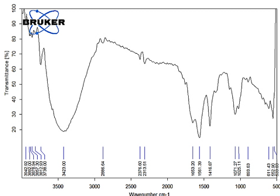
Gambar 4. Hasil analisis FTIR pada penggunaan NaOH 60%
