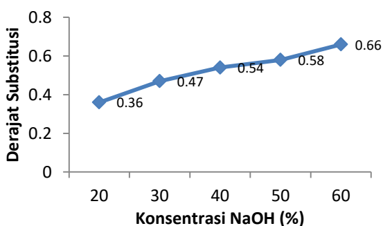
Gambar 3. DS O-KMK pada berbagai konsentrasi NaOH
