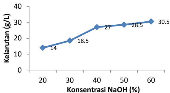
Gambar 2. Kelarutan O-KMK pada berbagai konsentrasi NaOH
