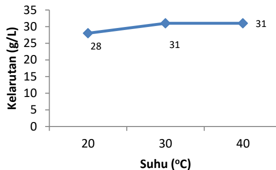
Gambar 6. Kelarutan O-KMK pada berbagai suhu
