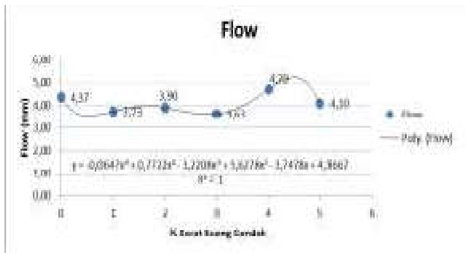
Gambar 5: Hubungan Flow Dengan Kadar Selulosa
