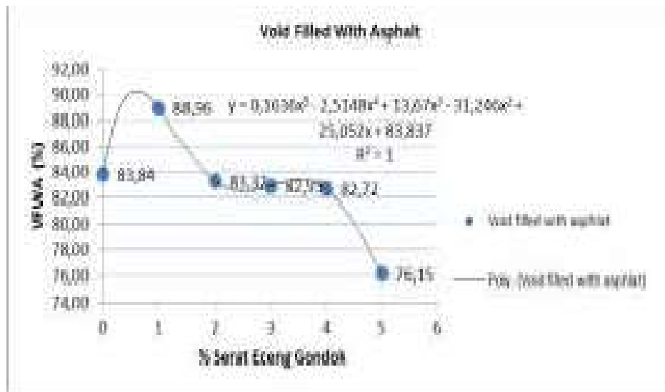
Gambar 4: Hubungan Void Filled With Asphalt Dengan Kadar Selulosa
