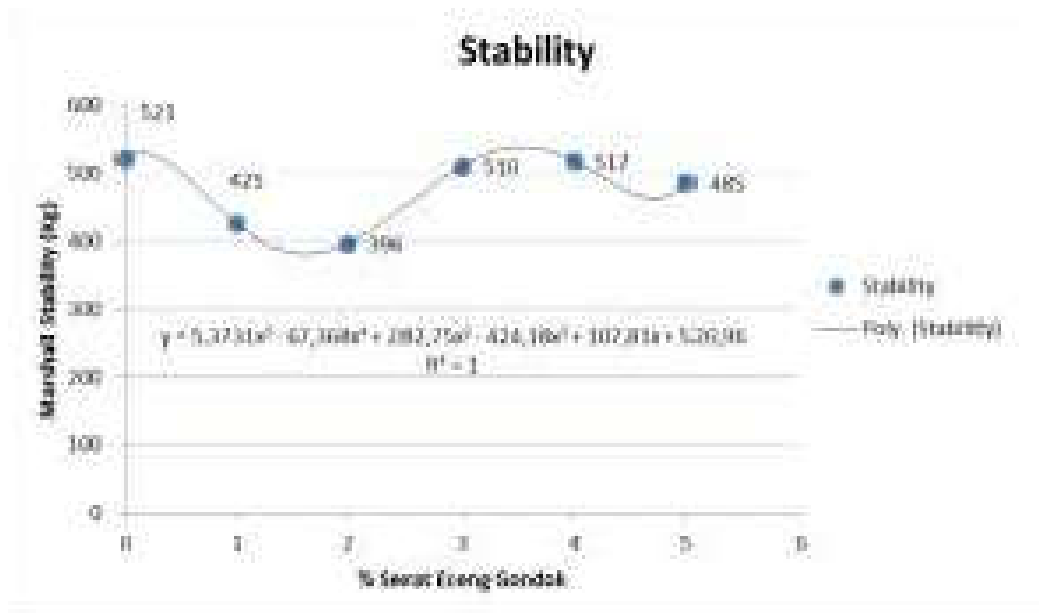
Gambar 1: Hubungan Marshall Stability Dengan Kadar Selulosa
