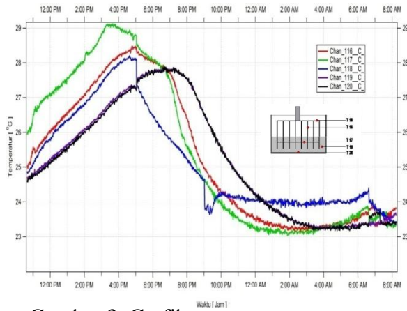
Gambar 3. Grafik temperatur evaporator vs waktu untuk temperatur pemvakuman 100°C dengan refrigerant (methanol)
