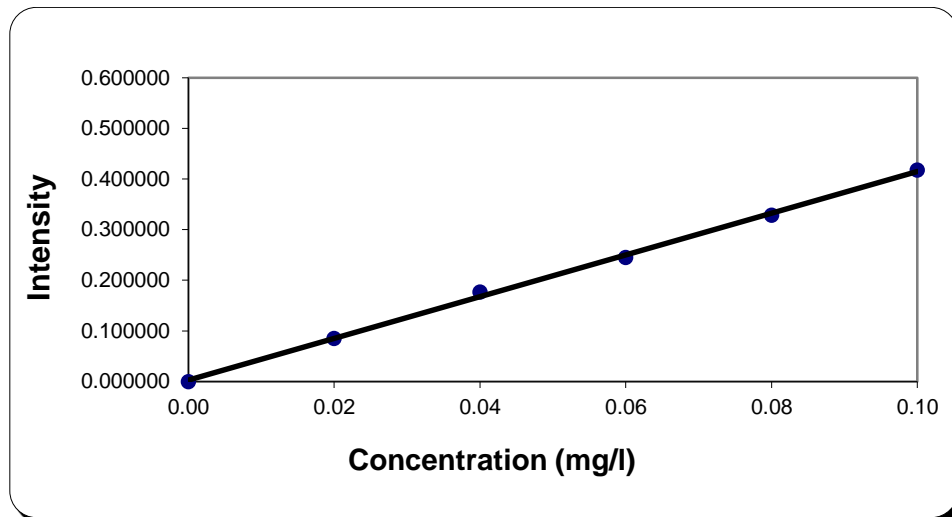
Gambar 1. Kurva kalibrasi antara serapan dengan beberapa konsentrasi standar Hg
