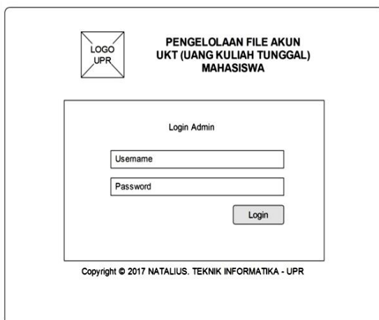
Gambar 4.5 Halaman Login
