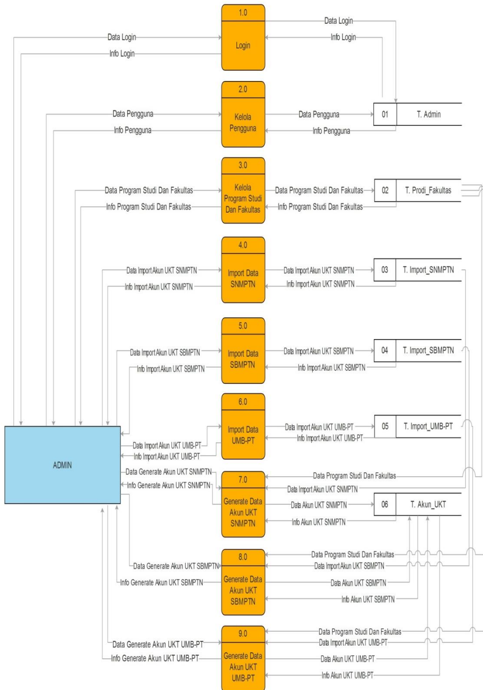
Gambar 4.2 DFD Level-1
