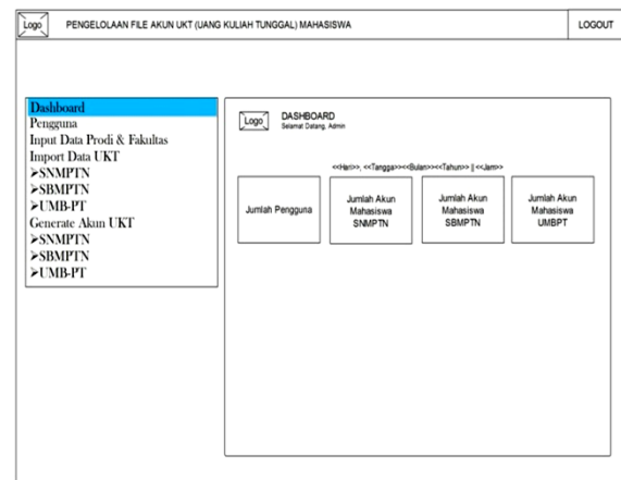
Gambar 4.6 Halaman Beranda
