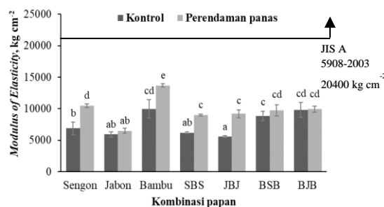
Gambar 6 Nilai MOE papan partikel hibrida dengan dan tanpa perlakuan perendaman panas; huruf yang sama menunjukkan tidak berbeda nyata ( \alpha < 0,5 ).
