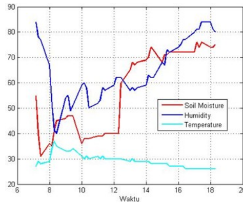
Gambar 9. Tampilan hasil perekaman sensor DHT11 dan Soil moisture secara Real Time
